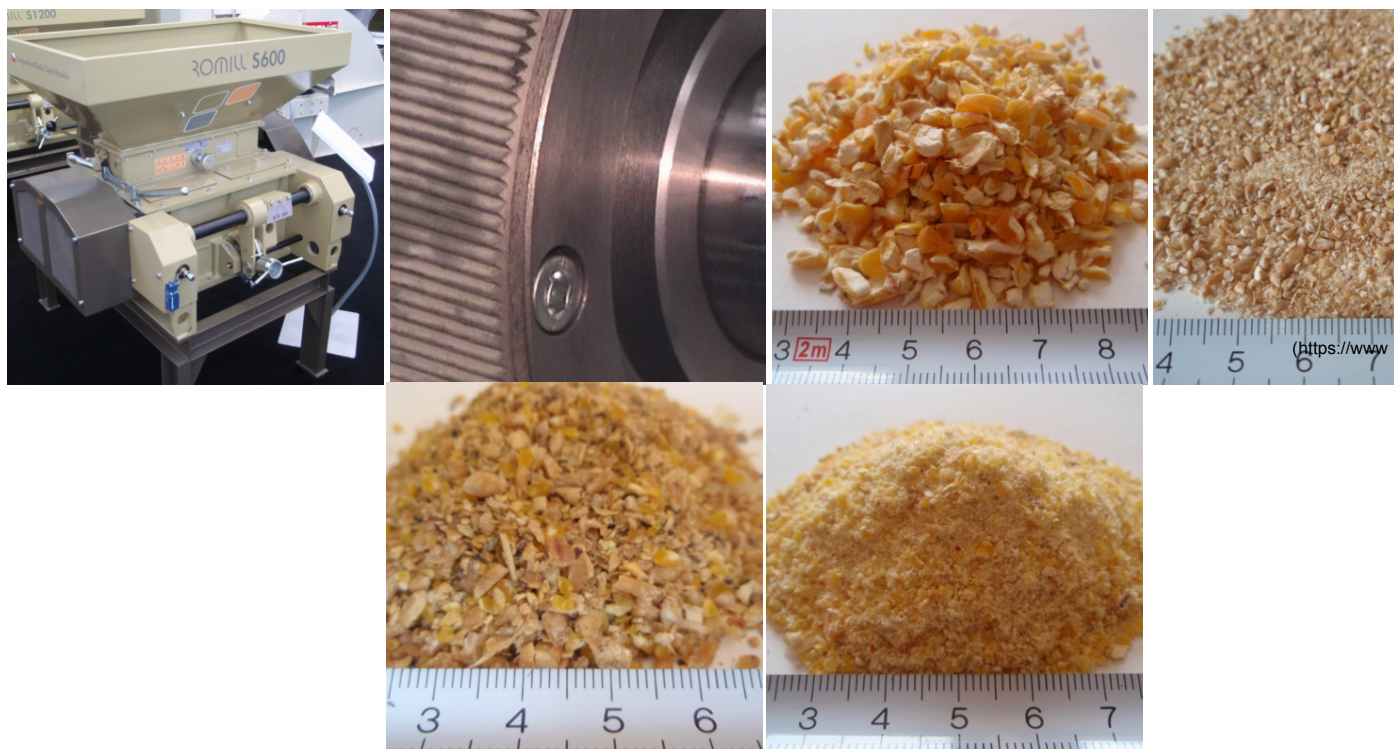
Стационарная вальцовая дробилка S600
